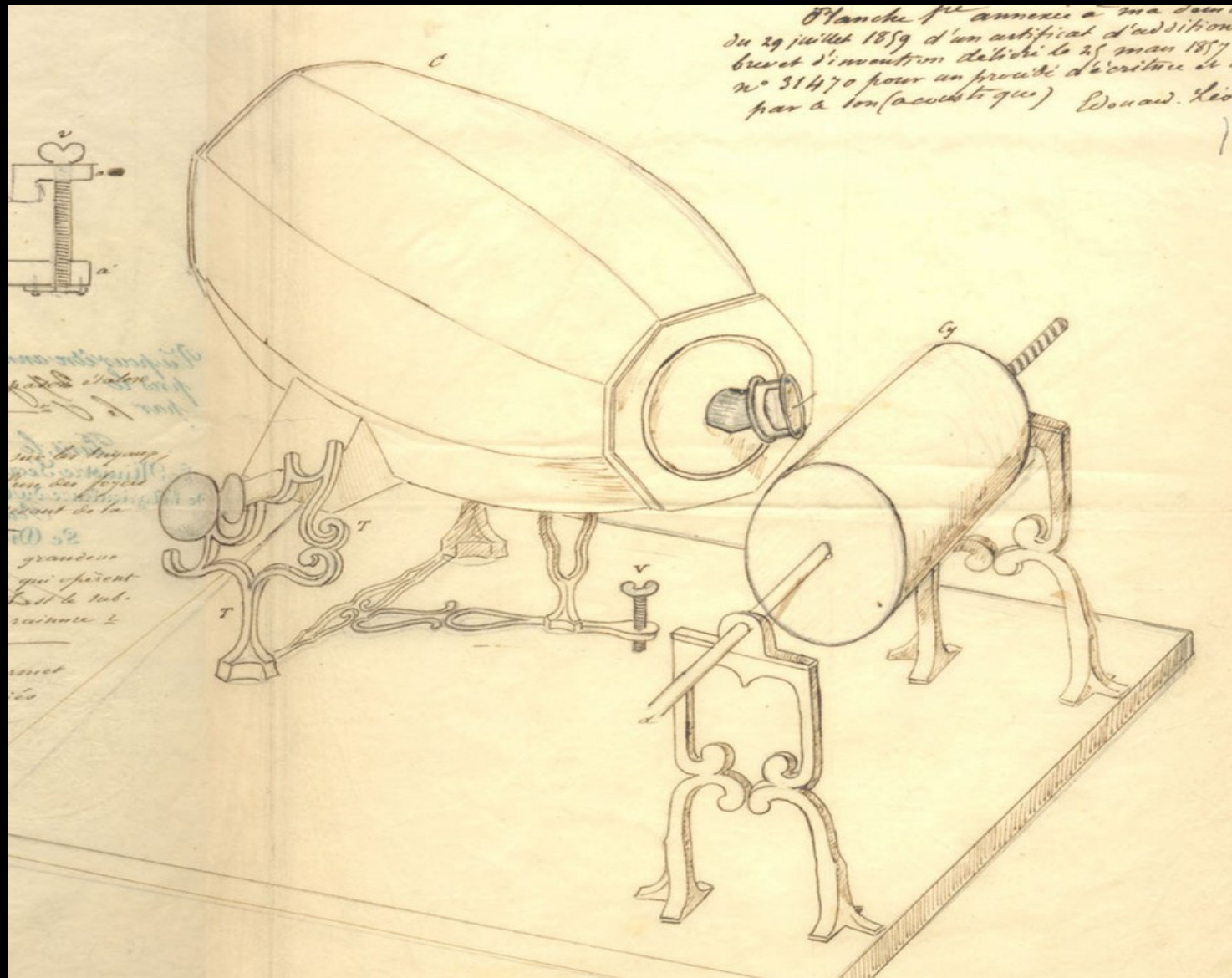
Édouard-Léon Scott de Martinville, Phonautographe , dessin du certificat d'addition (1859) au brevet d'invention. n° 17897 / 31470, INPI.
